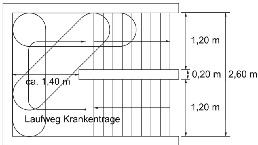
Abbildung 1: Mindestplatzbedarf einer Krankentrage, inkl. zwei Einsatzkräften (Träger)
