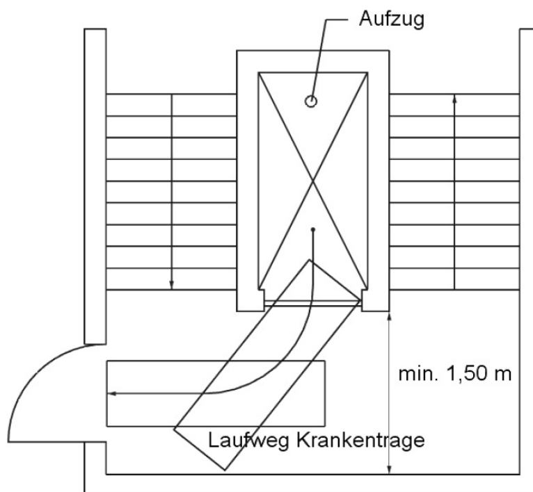
Abbildung 3: Exemplarische Darstellung eines Krankentransportes über einen Aufzug und dem notwendigen Platzbedarf vor dem Aufzug (nach DIN 18040)
