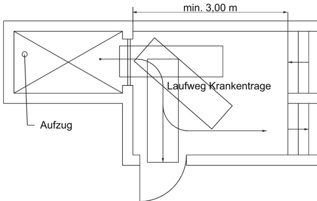
Abbildung 4: Exemplarische Darstellung eines Krankentransportes über einen Aufzug mit direkt gegenüberliegender Treppe und dem notwendigen Platzbedarf vor dem Aufzug (nach DIN 18040)
